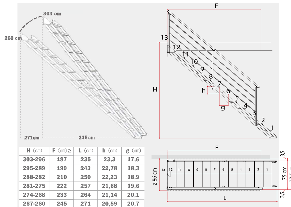
高さ寸法と平面寸法
